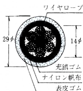
B-3.5T断面
