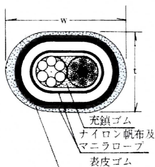
B-5T, 8T断面
