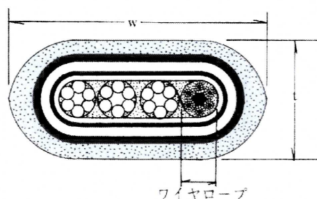
C-9T～25T断面・B-12T～25T断面
